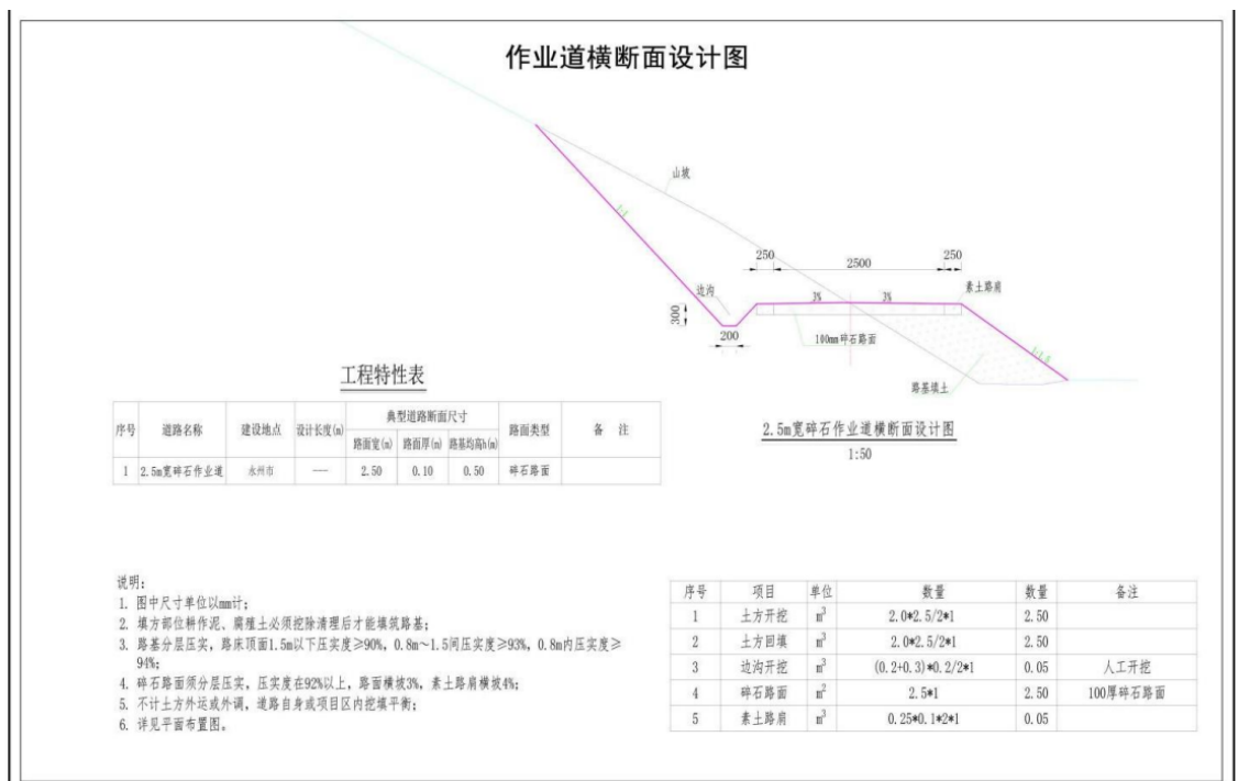
图 7-1 作业道横断面设计图
